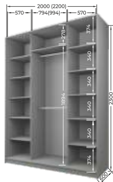
МШ-23-6-20/2-... МШ-23-6-22/2-...
