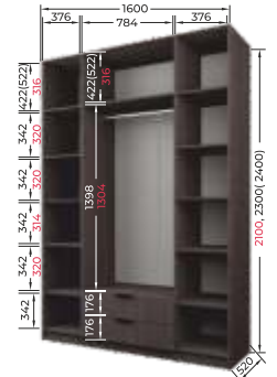
ЭШЗ-РП-21-16-2я ЭШЗ-РП-23(24)-16-2я
