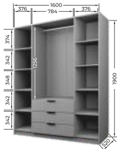
ЭШЗ-РП-19-16-3я
