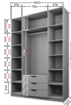
ЭШЗ-РП-21-16-3я ЭШЗ-РП-23(24)-16-3я
