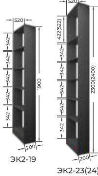
ЭК2-23(24)
