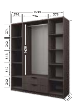
ЭШЗ-РП-19-16-2я
