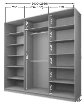
МШ-23-6-24/2-... МШ-23-6-27/2-...
