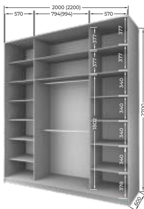
МШ-27-6-20/2-... МШ-27-6-22/2-...
