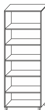
HШР-1-2-5 В x Ш x Г 2140x800x520
