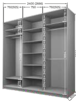
МШ-23-6-24-... МШ-23-6-27-...
